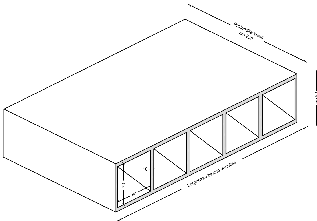
ASSONOMETRIA
